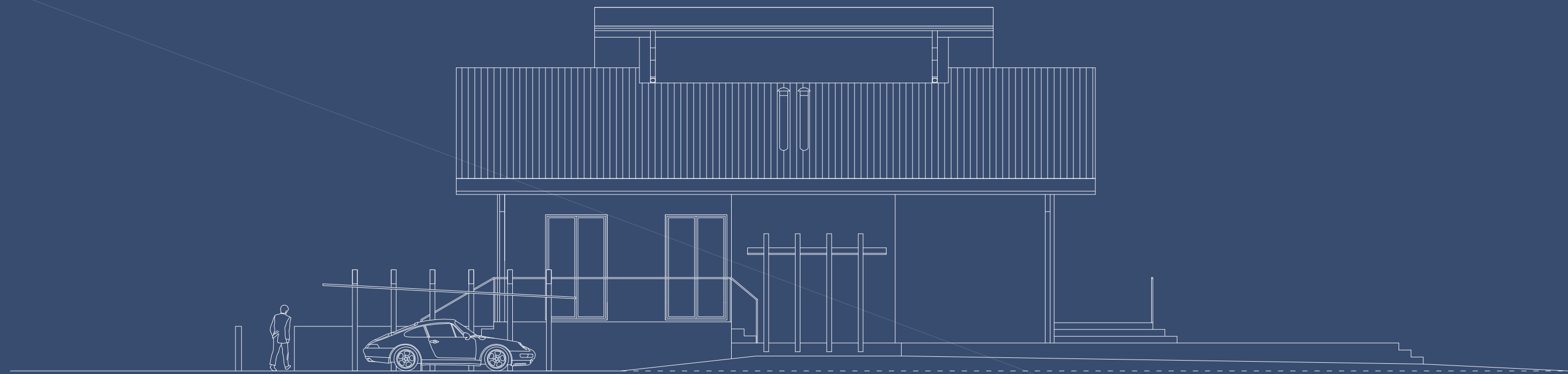
PROSPETTO SUD
